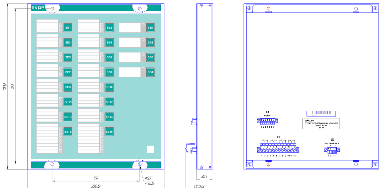
Рисунок 1 – Общий вид и габаритные размеры пульта электронных ключей У1140
